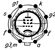
Sockelschaltenschema
